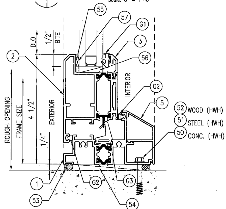
1 STANDARD SILL (OUT-SWING) Scale: 6" = 1'-0"
