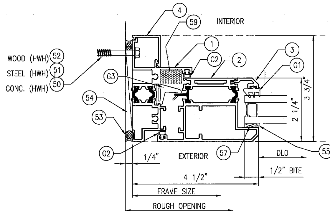
4 JAMB (OUT-SWING) Scale: 6" = 1'-0"
