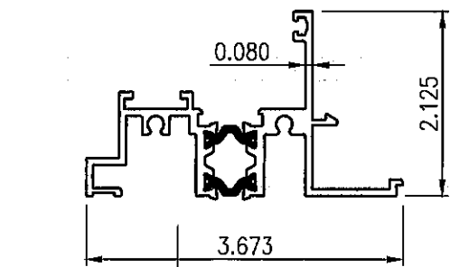
1 SUN-4113 FRAME Scale: 6" = 1'-0"
