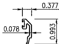
3 SUN-4119 GLAZING BEAD Scale: 6" = 1'-0"
