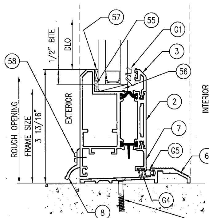
3 ADA SILL (OUT-SWING) Scale: 6" = 1'-0"
