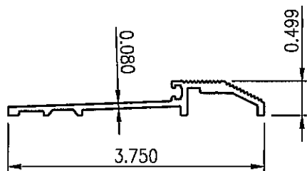
6 SUN-4100 ADA THRESHOLD Scale: 6" = 1'-0"
