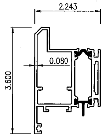
1 SUN-4113 FRAME Scale: 6" = 1'-0"
